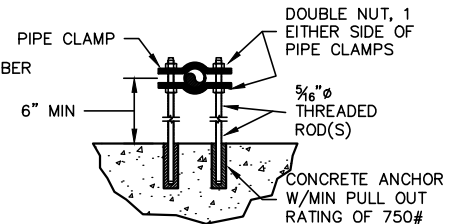
PIPE CLAMP (WALL)
